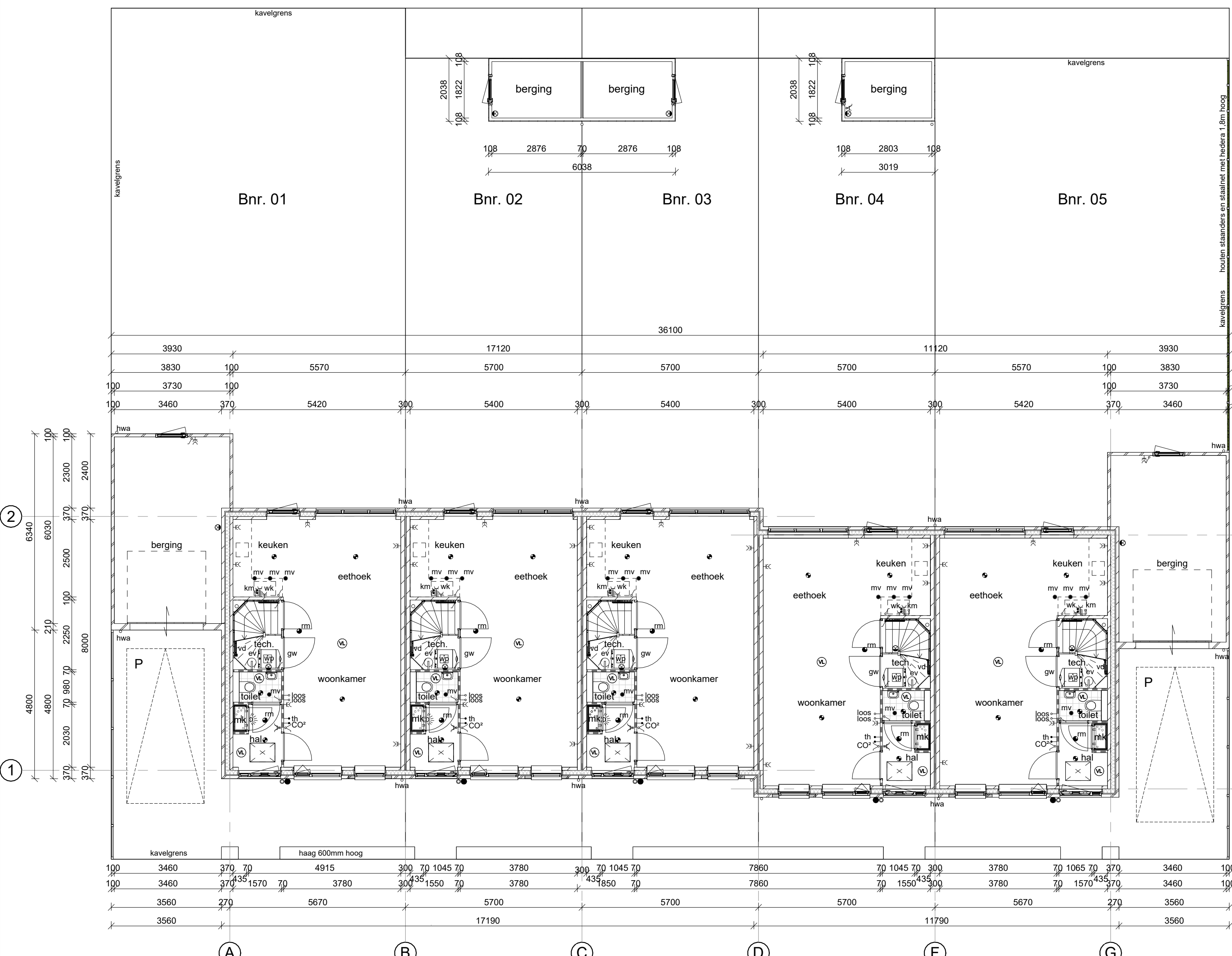
begane grond
