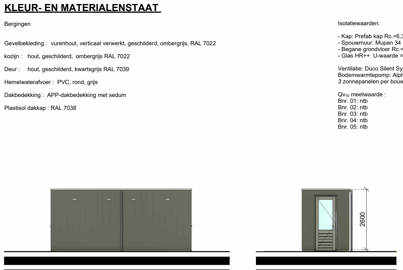
vooraanzicht
