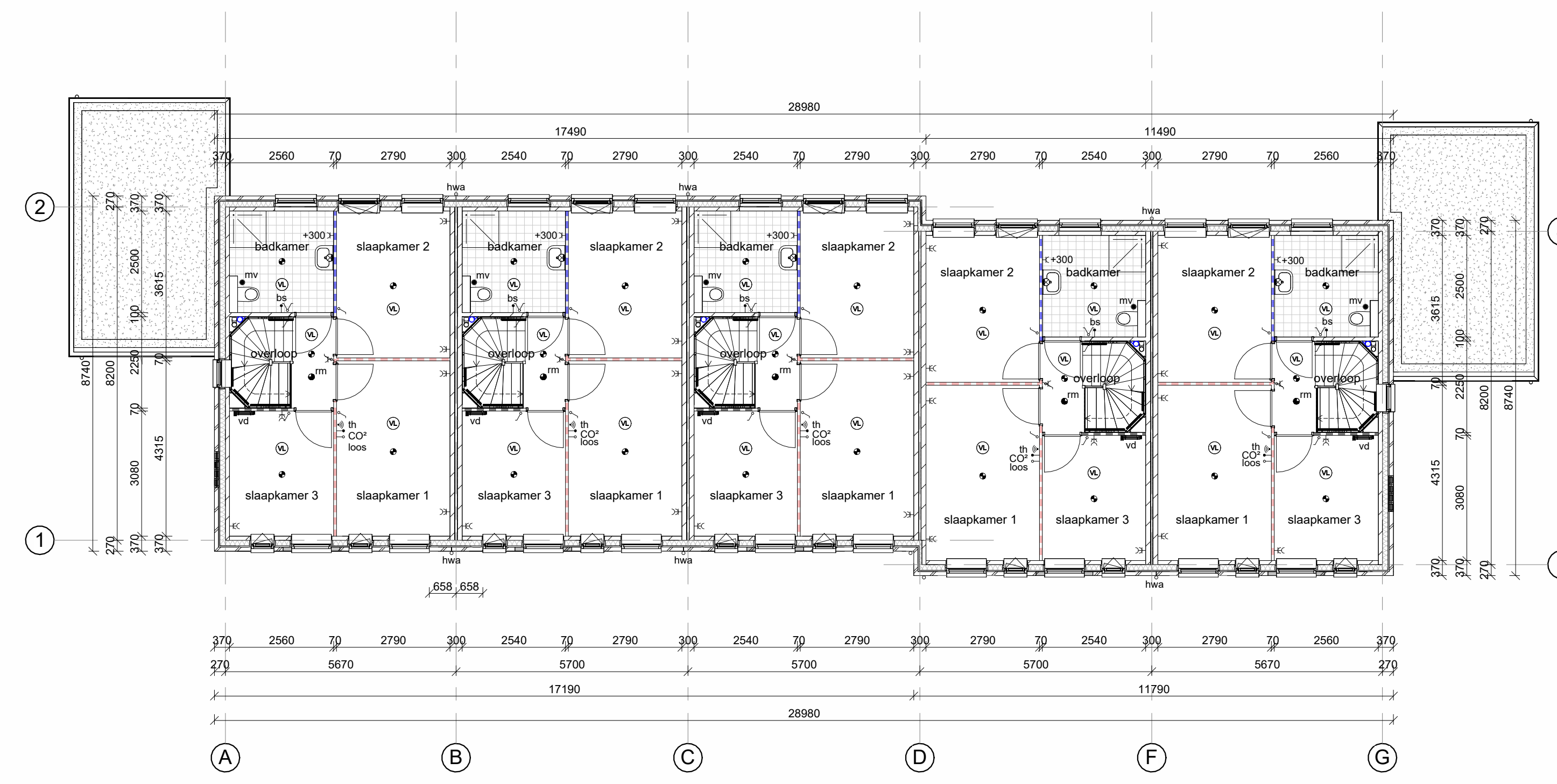
1e verdieping
