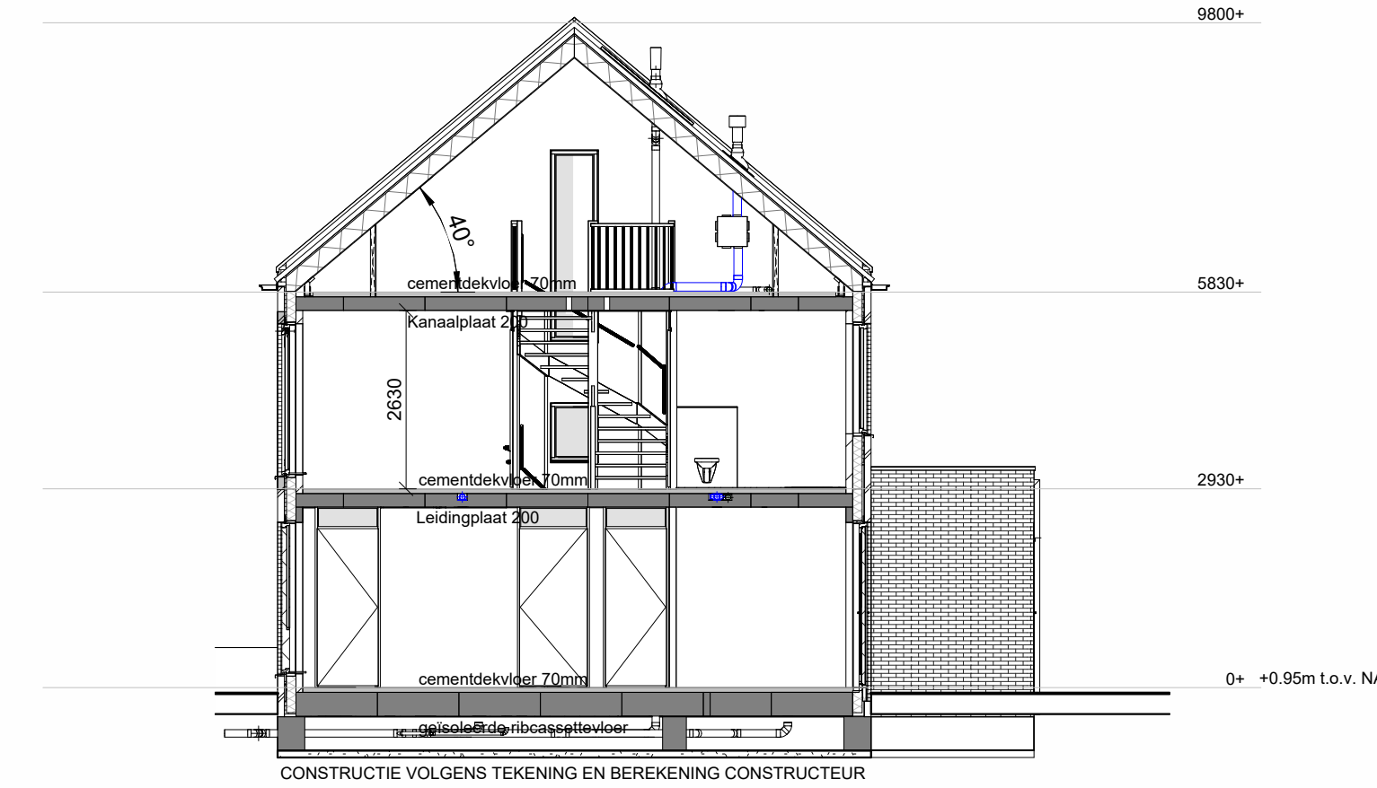
doorsnede
