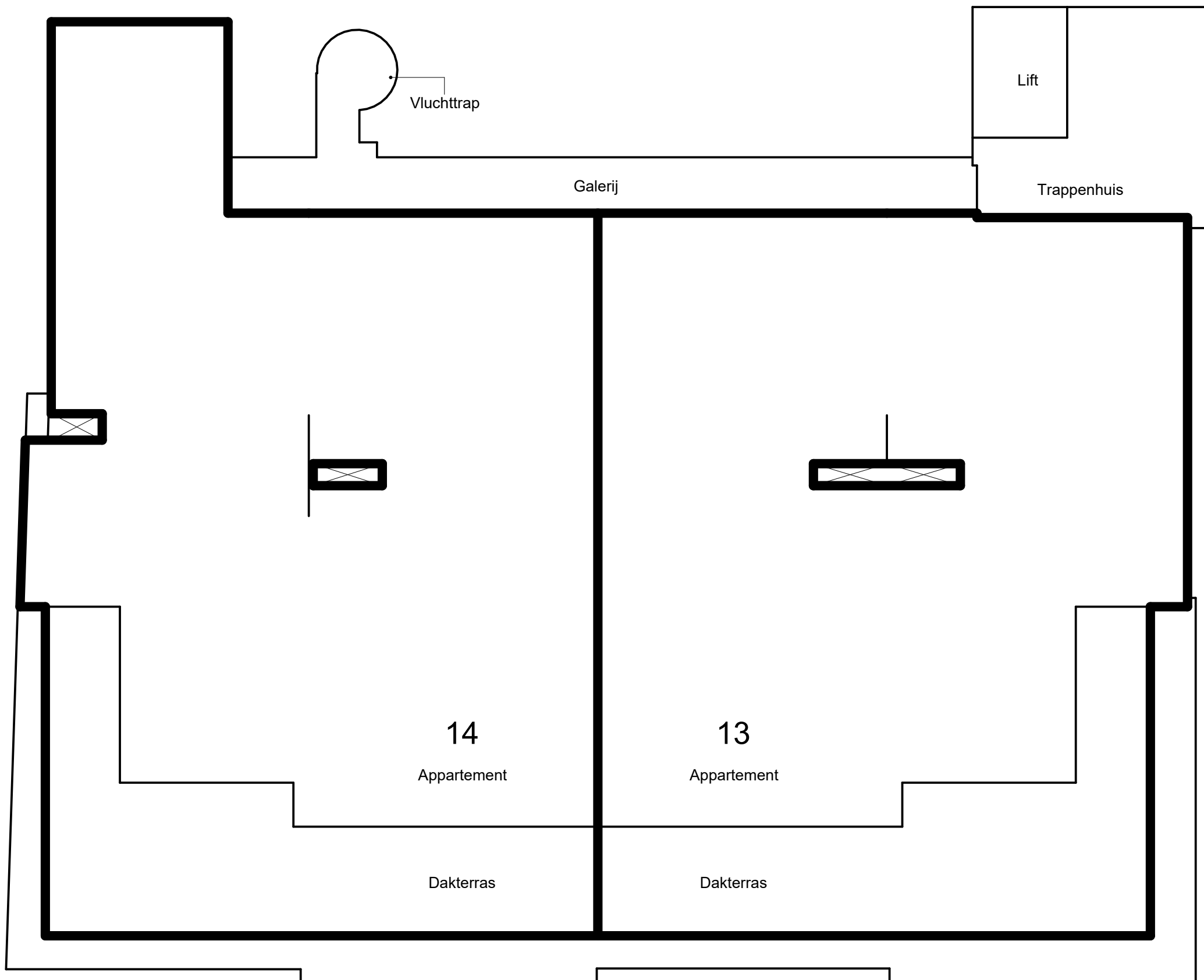
4e VERDIEPING
