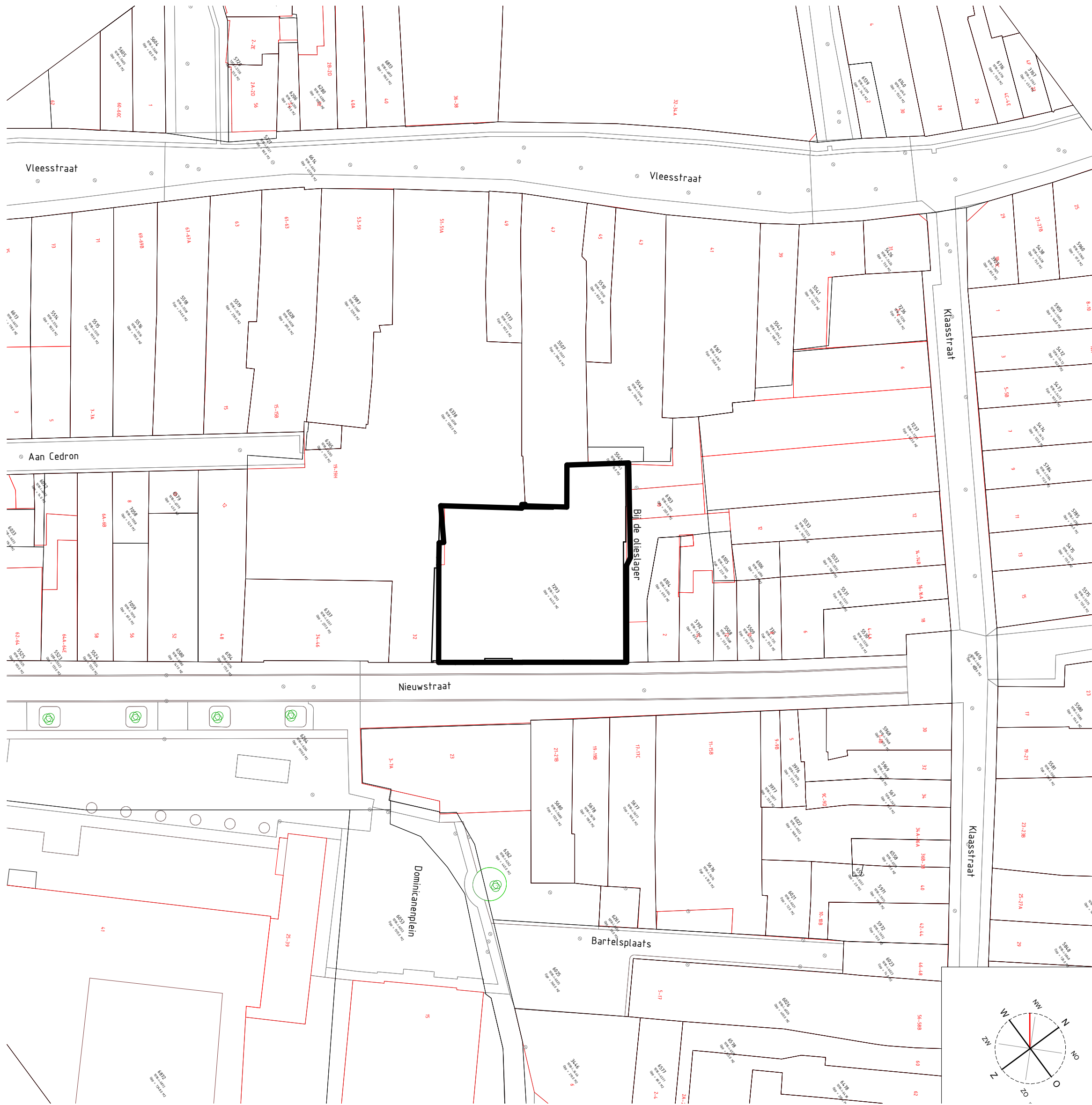
Situatie
