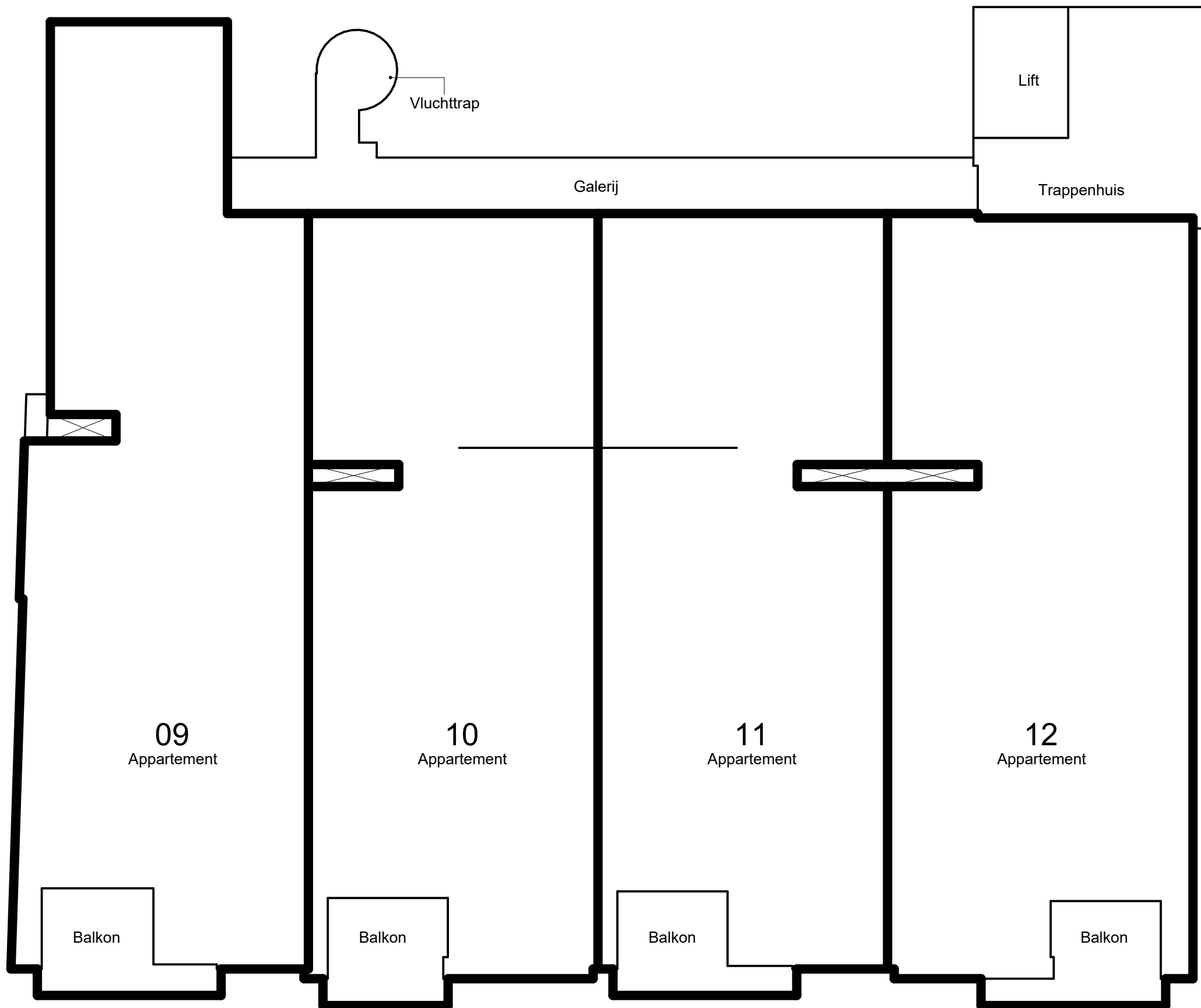
3e VERDIEPING
