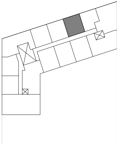
10.11 10e verdieping
