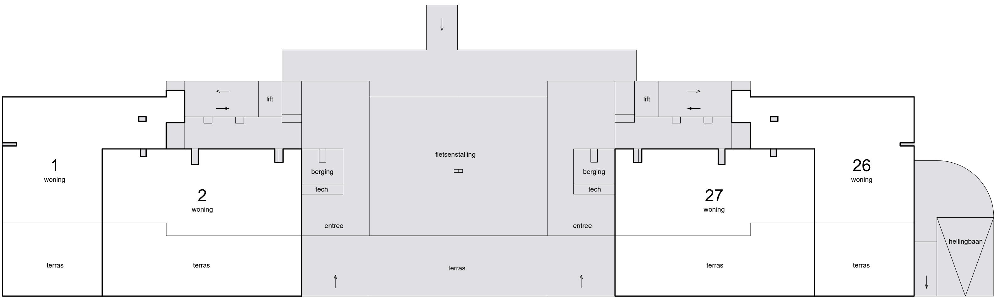
begane grond
