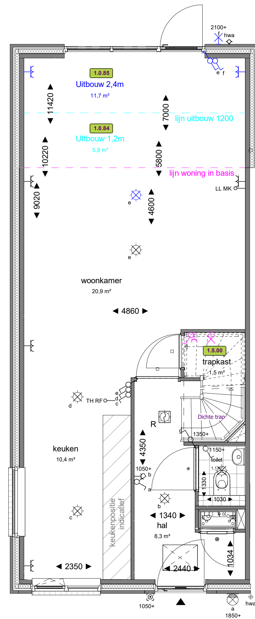
Rij-5100 Uitbouw 1200/2400 en trapkast Schaal: 1 : 50 van toepassing bij Bnr 15-18-25-30
