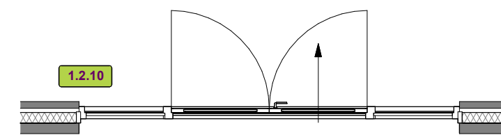
Rij-5100 vergrote zijlichten bij openslaande deuren
