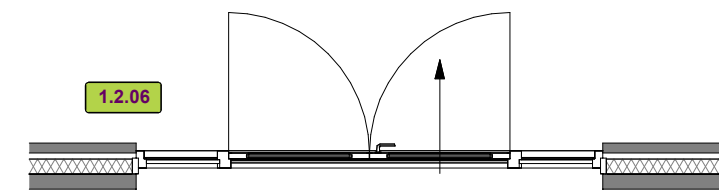
Rij-5100 openslaande dubbele deuren
