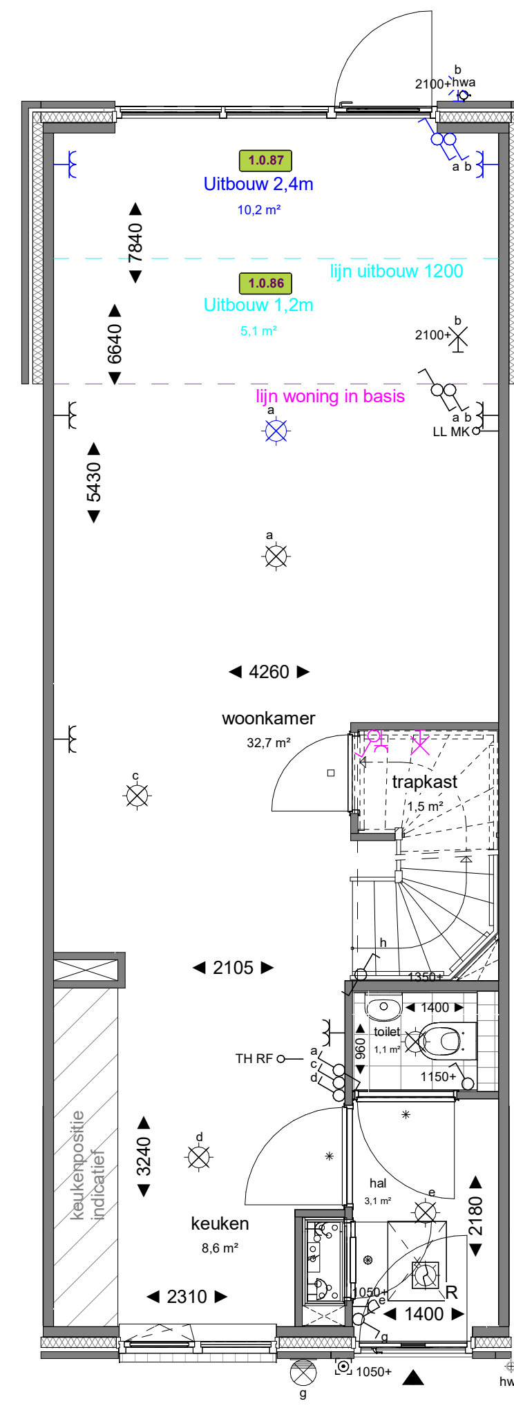
Rij-4500 Uitbouw 1200/2400 en trapkast Schaal: 1 : 50 van toepassing bij Bnr 16-17-18-26-27-29
